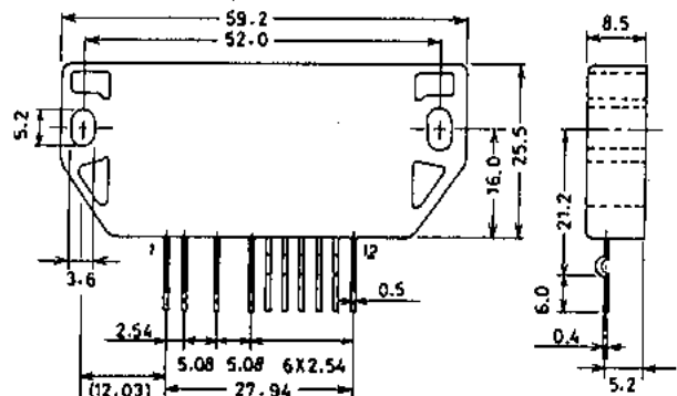
外形図 4055 (unit:mm)
